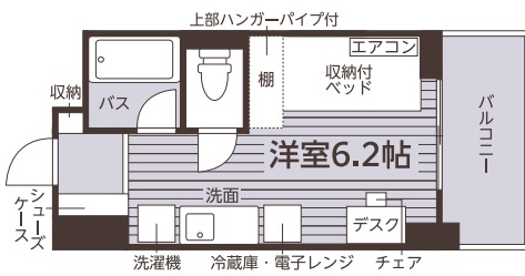
E 1Rタイプ (15.7㎡)
