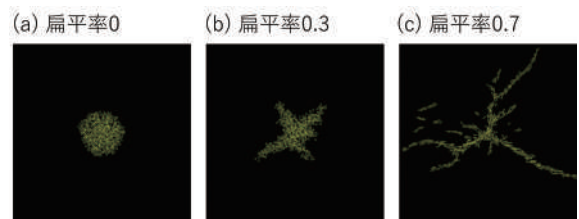
図2:血管網形状の楕円扁平率依存性
