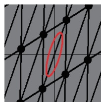
図3b 斜め方向に引っ張られたグラフ
