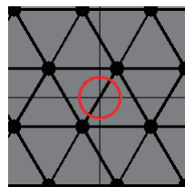
図3a 等方的なグラフ
