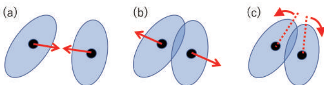
図1:細胞間の2体相互作用。(a)細胞間引力:接着性分子による効果、(b)排除体積効果による近距離斥力:物質が空間を占有する効果、(c)接触による回転:重なりを避ける向きへの回転
