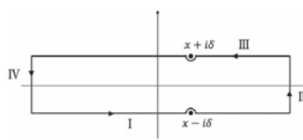
Fig.2: coth型特異積分核に対応する複素領域
