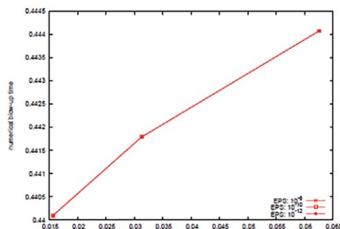
図2 数値爆発時間
