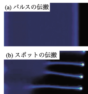
図3 数値計算結果
