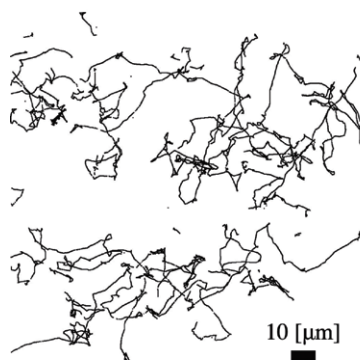
図1 個々の大腸菌の軌跡
