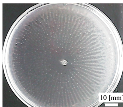
図2 大腸菌の集団的パターン
