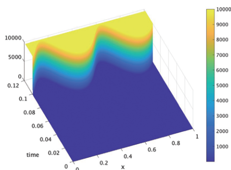
図1 非線形波動方程式の爆発解
