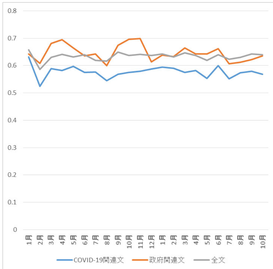
図 10 daigo/bert の分析結果（時系列）
